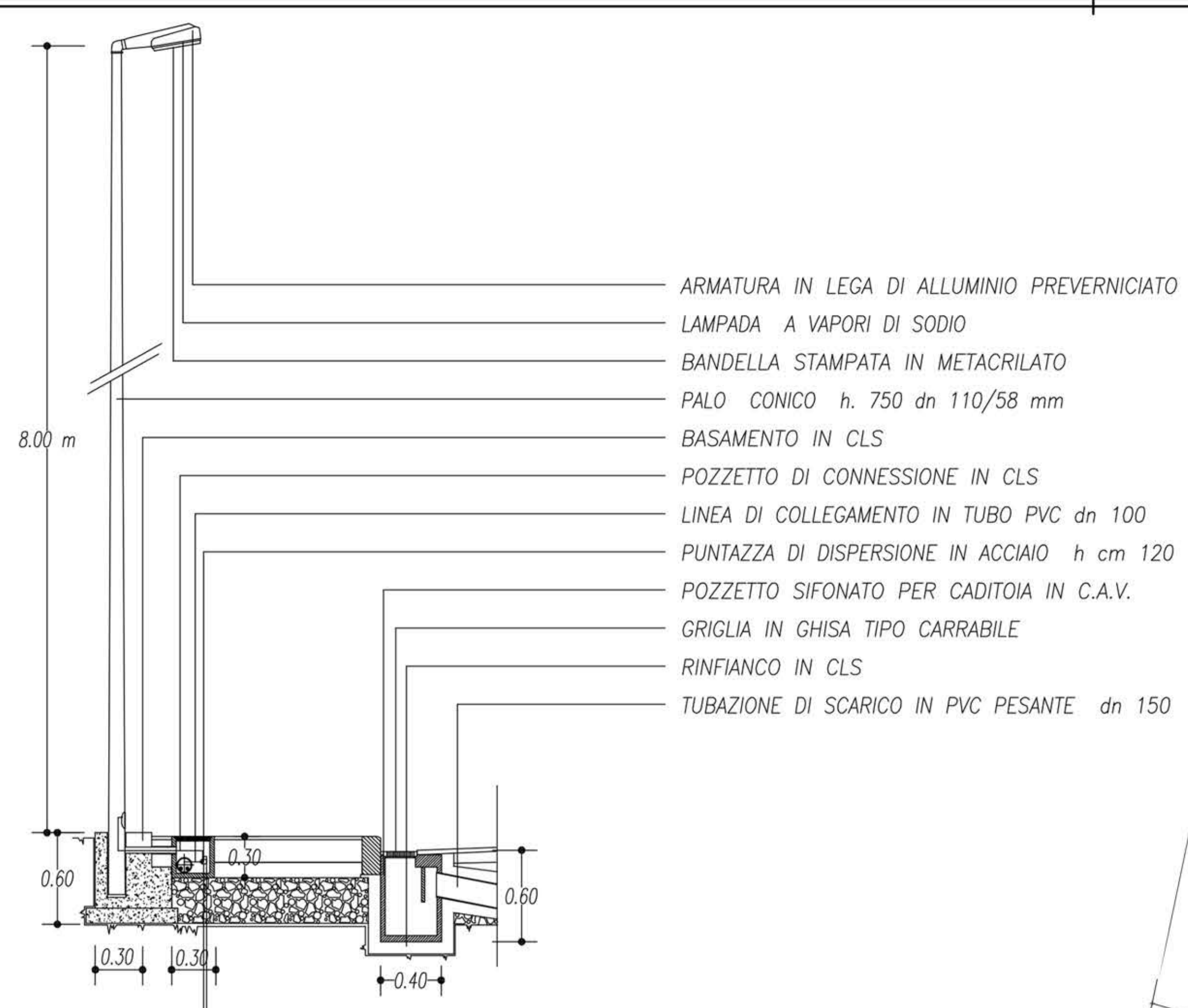
LAMPIONE PER ILLUMINAZIONE STRADALE E PARCHEGGI PUBBLICI SCALA 1: 50
